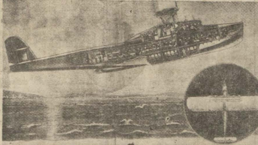
Tayyarenin iç tertibatı
